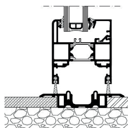
Lodret snit - med bundskinne i reces
