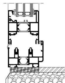
Lodret snit - med anslagskarm
