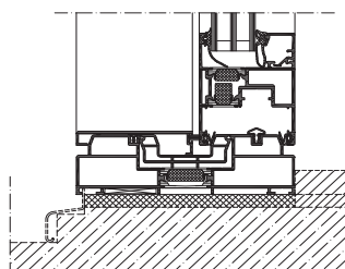
Tilslutningsprincip, hæve-skydesystem
