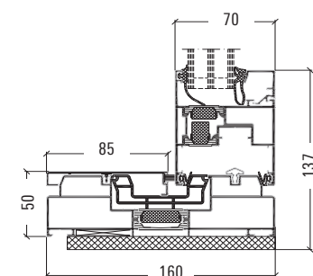
Profilmål, hæve-skydeparti
