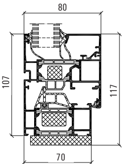
Profil mål, vindue
