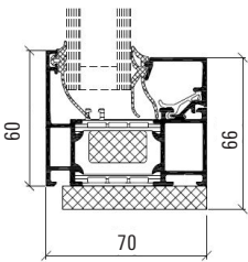
Profil mål, vindue
