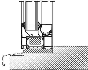
Tilslutningsprincip, fast felt
