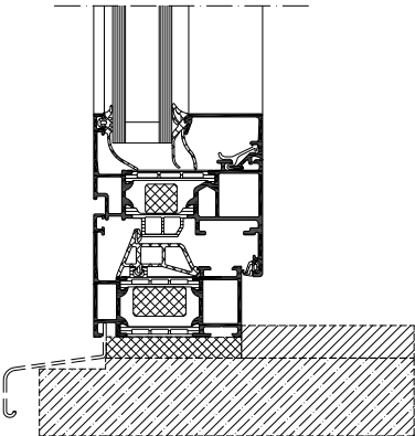
Tilslutningsprincip, vindue
