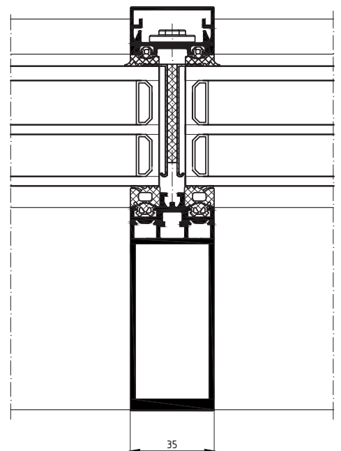
Schüco facadesystem FWS 35 PD
